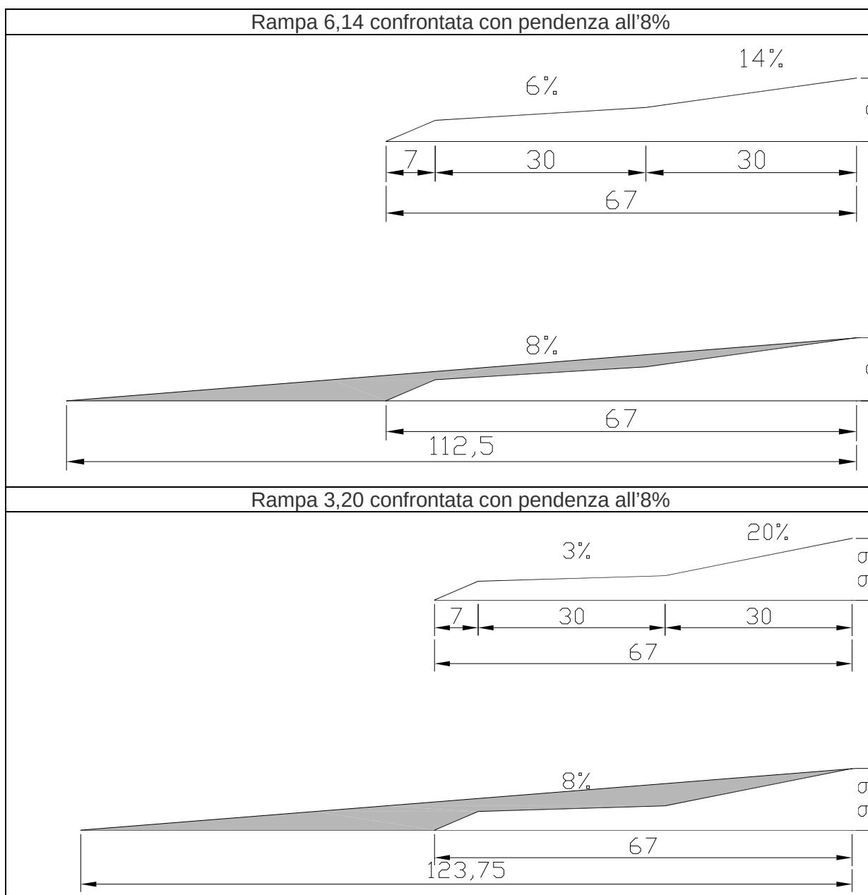
Fig. 7_ Confronto tra rampa a gradino agevolato e rampa tradizionale
